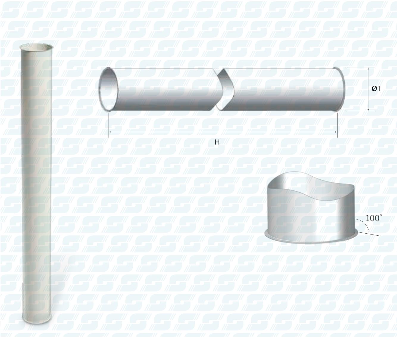
Tubazioni H.2000 con bordo - Straight pipe H 2000 with flared end
